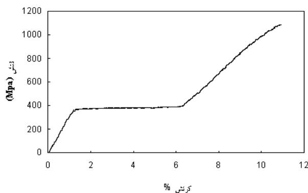
شکل ۶- منحنی تنش-کرنش سیم خام تا نقطه شکست.
