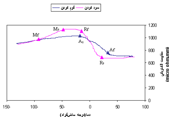
شکل ۴- منحنی تغییرات رسانایی الکتریکی بر حسب دما.
