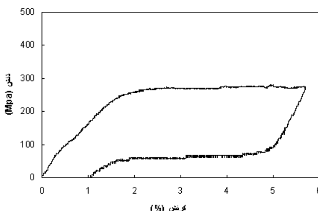
شکل ۹- منحنی تنش-کرنش سیم در اثر عبور جریان الکتریسیته ۴/۵ آمپر.
