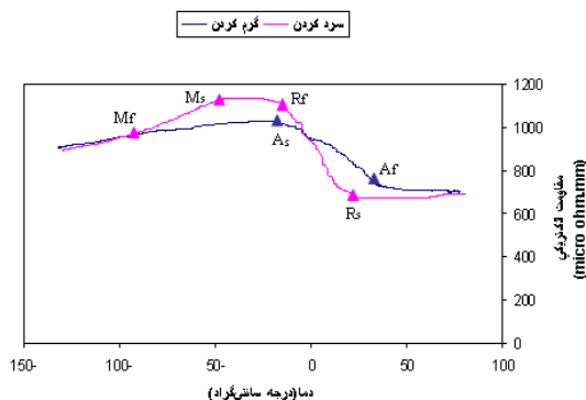
شکل ۴- منحنی تغییرات رسانایی الکتریکی بر حسب دما.
